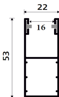
Guida 22x53 mm
