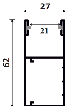
Guida 27x62 mm
