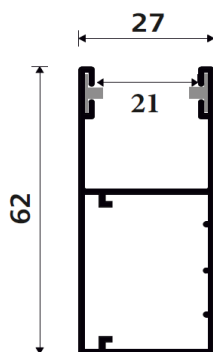
Guida 27x62 mm
